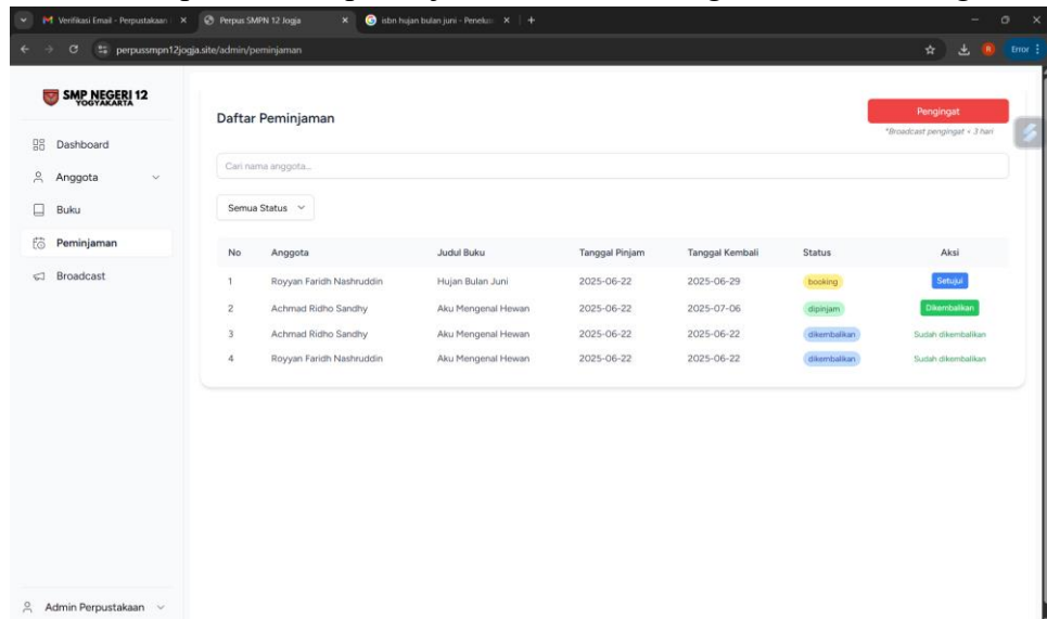
Gambar 18. Data Peminjam
