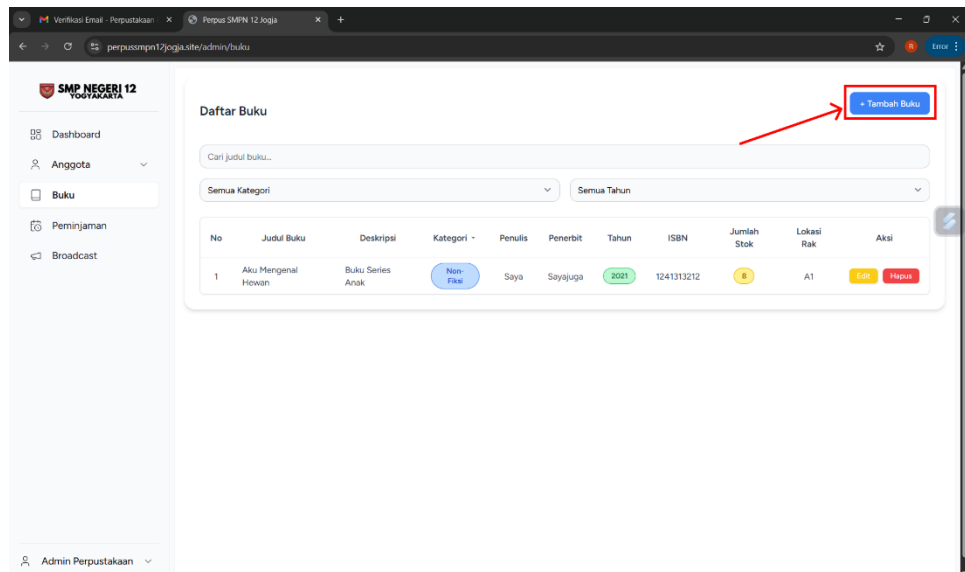
Gambar 13. Page Buku
