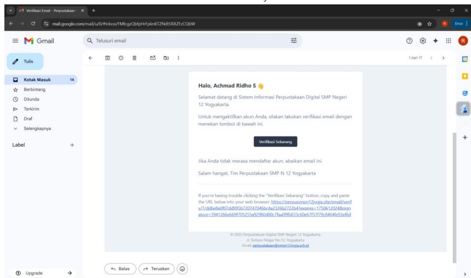
Gambar 31. Verifikasi email
