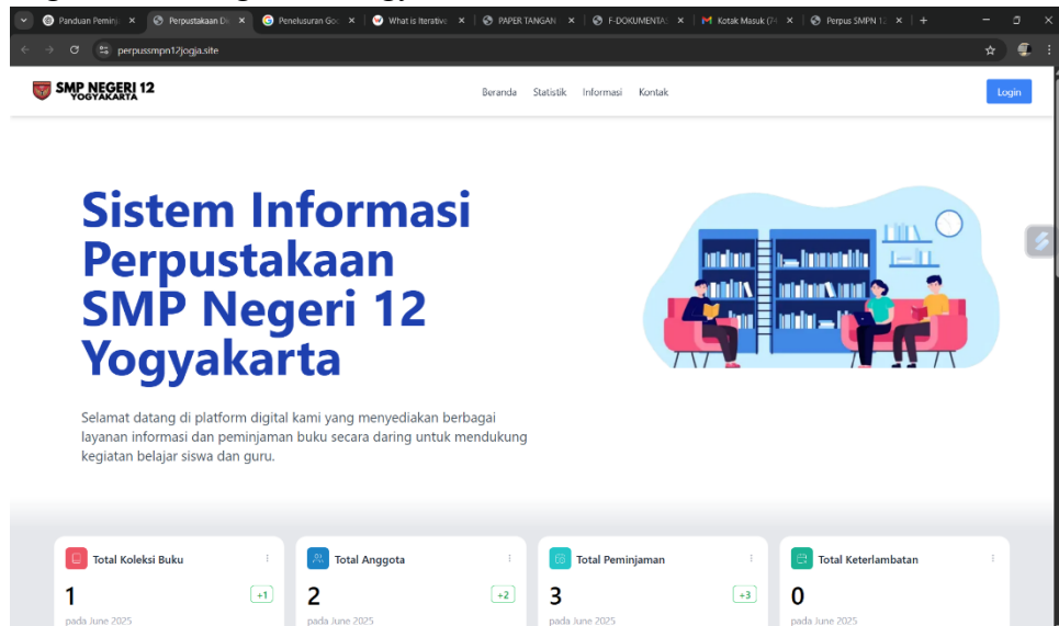
Gambar 26. Welcome Page
