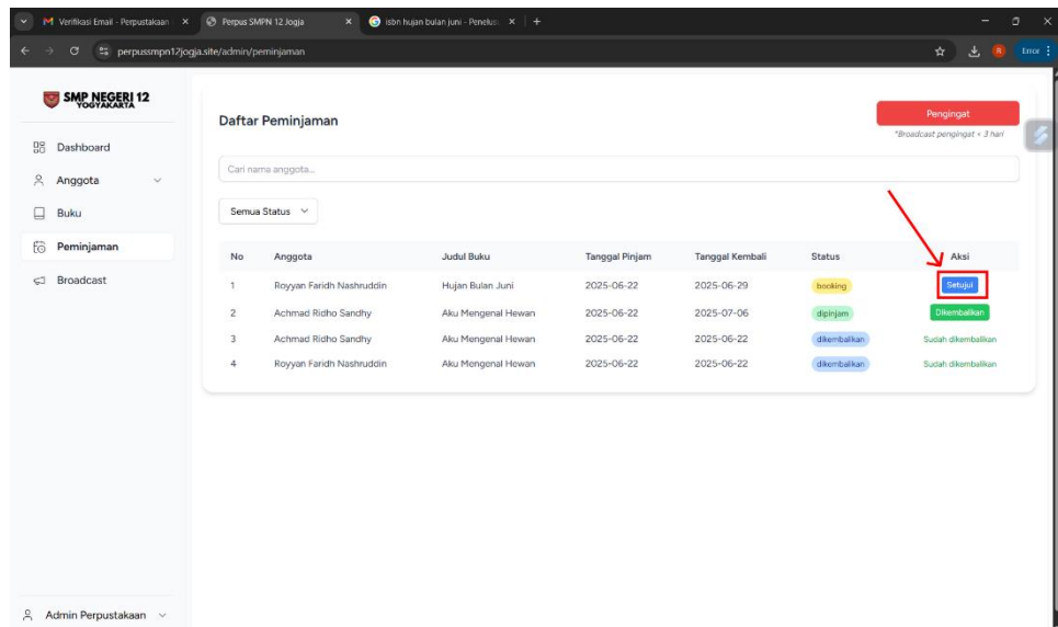
Gambar 19. Menyetujui Peminjaman
