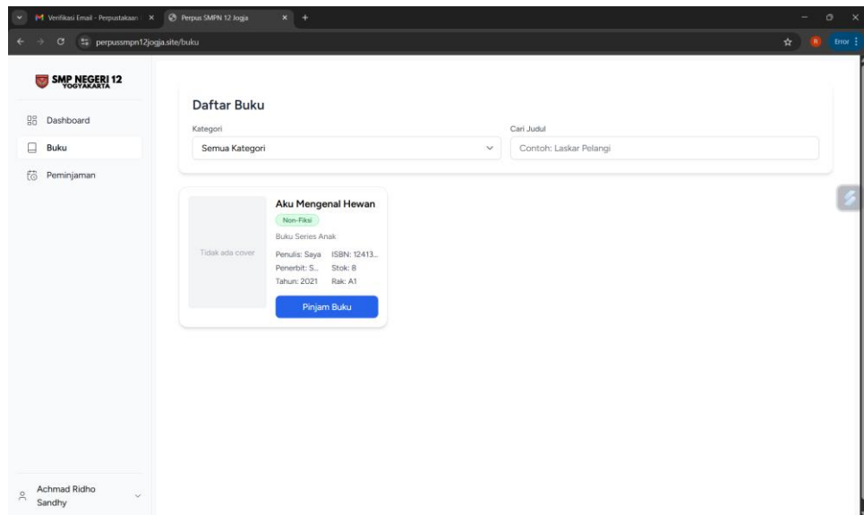
Gambar 34. Page Buku
