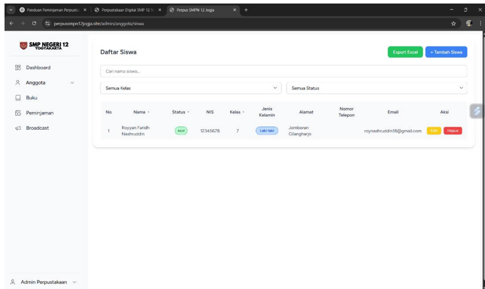
Gambar 7. Page Anggota
