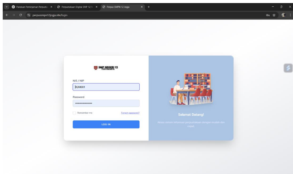
Gambar 4. Login Page
