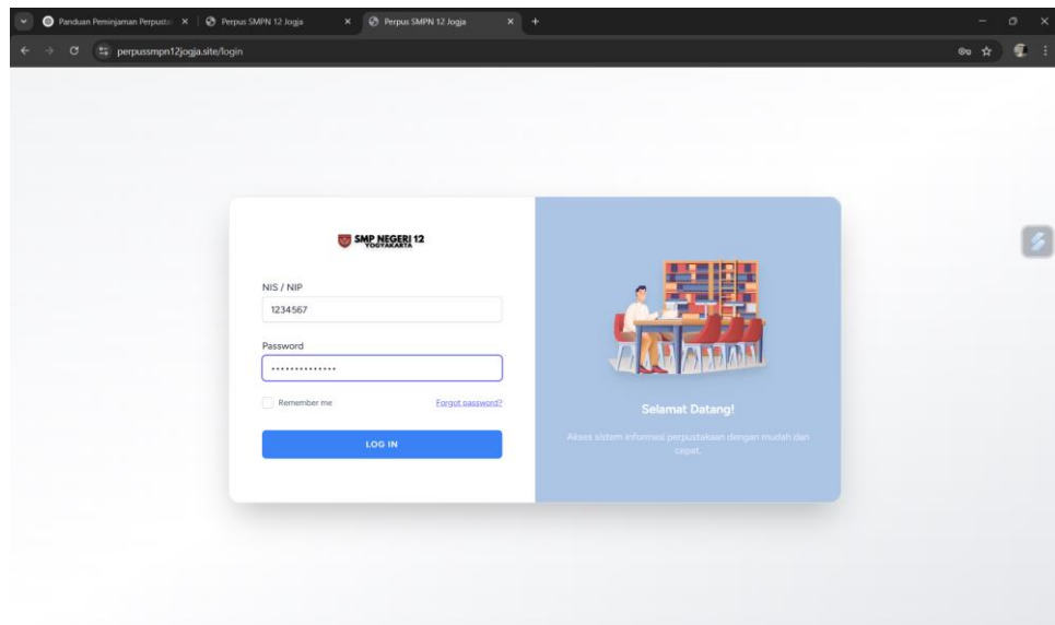
Gambar 28. Login Page
