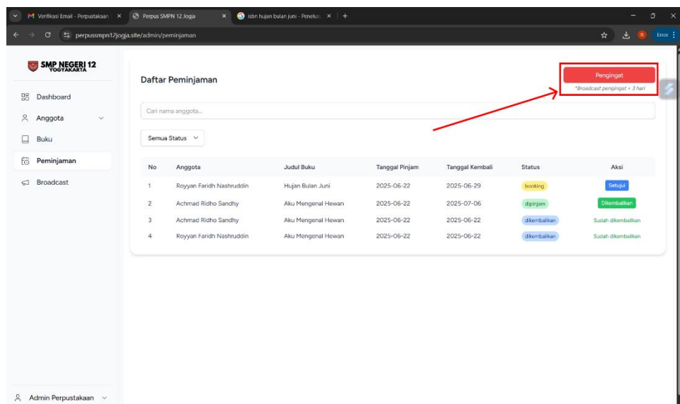
Gambar 20. Peringat peminjaman
