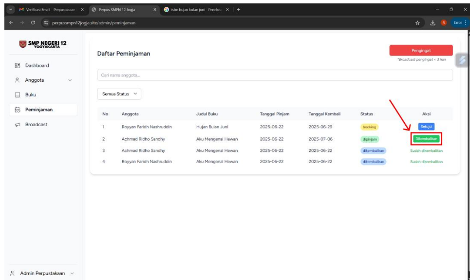
Gambar 21. Konfirmasi pengembalian
